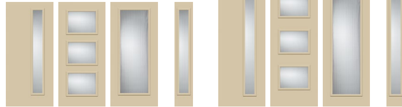
FS9531-R* FS9533 FS9591 FSS981 FS9531-R* FS9533 FS9591 FSS981 W: 2'6", 2'8", 2'10", 3'0" 2'8", 2'10", 3'0" 2'8", 2'10", 3'0" 12", 14", 16" 2'6", 2'8", 2'10", 3'0" 2'8", 2'10", 3'0" 2'8", 2'10", 3'0" 12", 14", 16" H: 6'8", 7' 6'8", 7' 6'8", 7' 6'8", 7' 8' 8' 8' 8'
